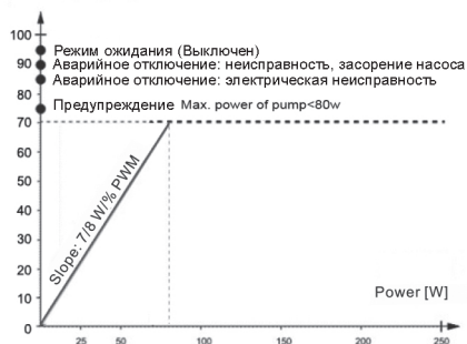
Рис 8. Логика сигнала обратной связи ШИМ
